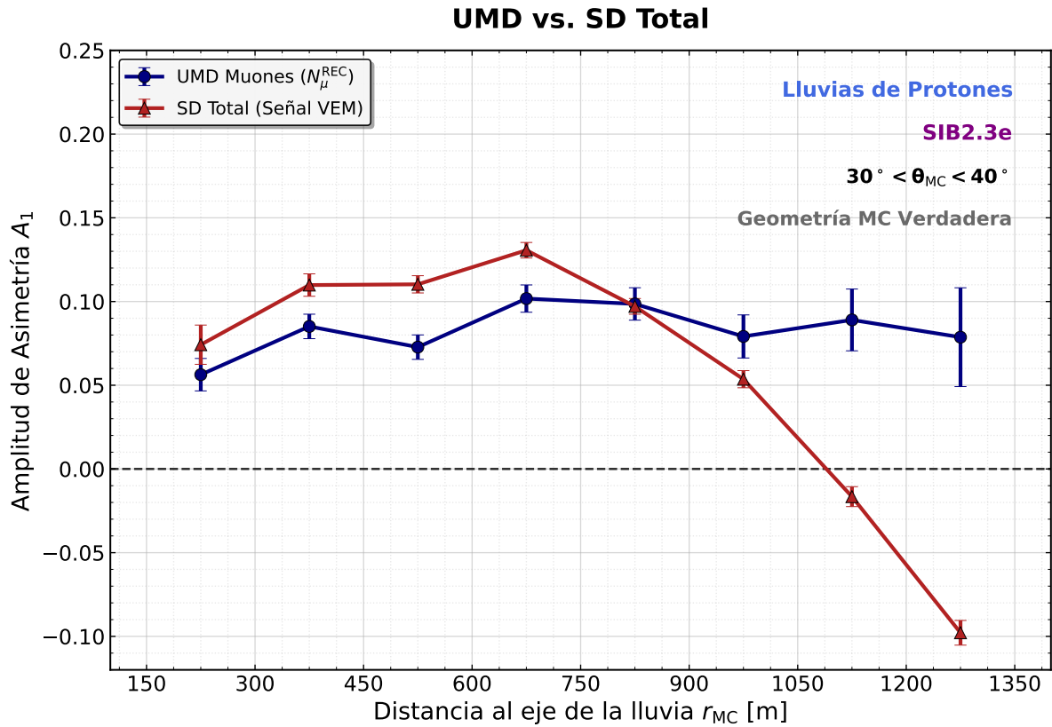
Figura 6.3: [caption modificado] Comparación de la evolución radial de la amplitud de asimetría A_1 entre el número de muones reconstruido por el UMD ( N_{\mu}^{REC} ) y la señal total registrada por los tanques del SD en superficie, evaluada para el rango cenital de referencia de 30^{\circ} \leq \theta < 40^{\circ} . Ambas curvas fueron extraídas fijando la geometría real de Monte Carlo; las barras de error representan el error estándar de la media. Se evidencia el comportamiento divergente de los observables: mientras que el UMD mantiene una asimetría positiva a todas las distancias, la señal del SD Total exhibe una severa disminución de la asimetría que culmina en una inversión (asimetría negativa) en el far-core .
